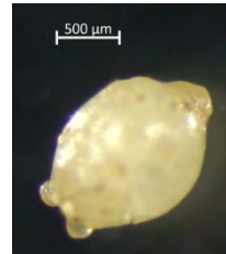
Semisolid syntetisk partikel från Munksjöns utlopp.
