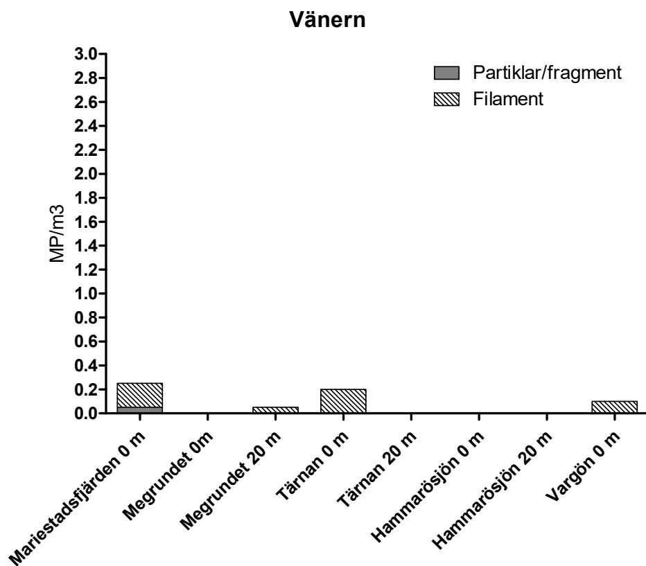
Figur 10. Sammansättning och antal mikroplaster > 300 µm (MP/m³) i proven från Vänern.
