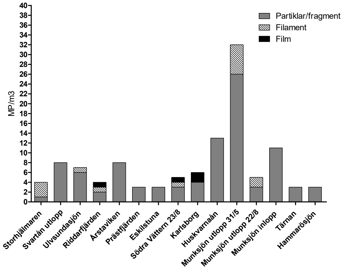
Figur 13. Sammansättning och antal mikroplaster (MP/m³) i 50-300 µm fraktionen i prov från samtliga sjöar med koncentrationer över rapporteringsgränsen 2 MP.
