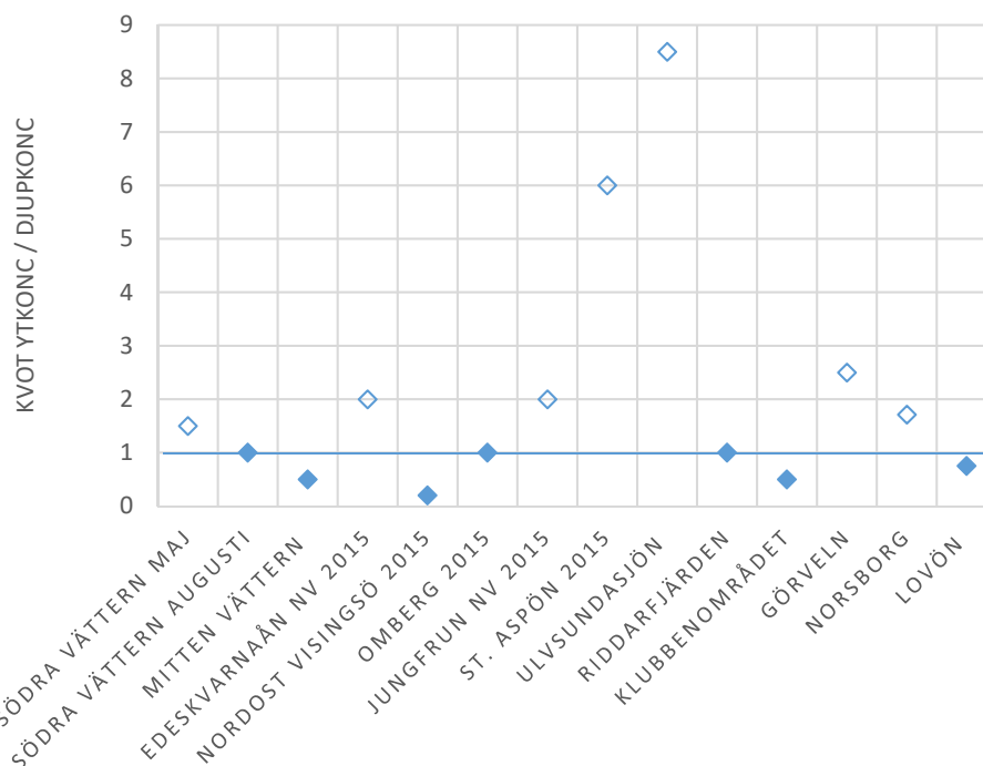
Figur 5. Kvot mellan mikroplastkoncentrationen i ytvatten (MP/m 3 ) (0 m) och i en djupzon (12-15 m i Ulvsundasjön, Klubbenområdet, Riddarfjärden och Vättern 2015, 20 m i Vättern 2017 och 22 m i Görväln och Lovön).
