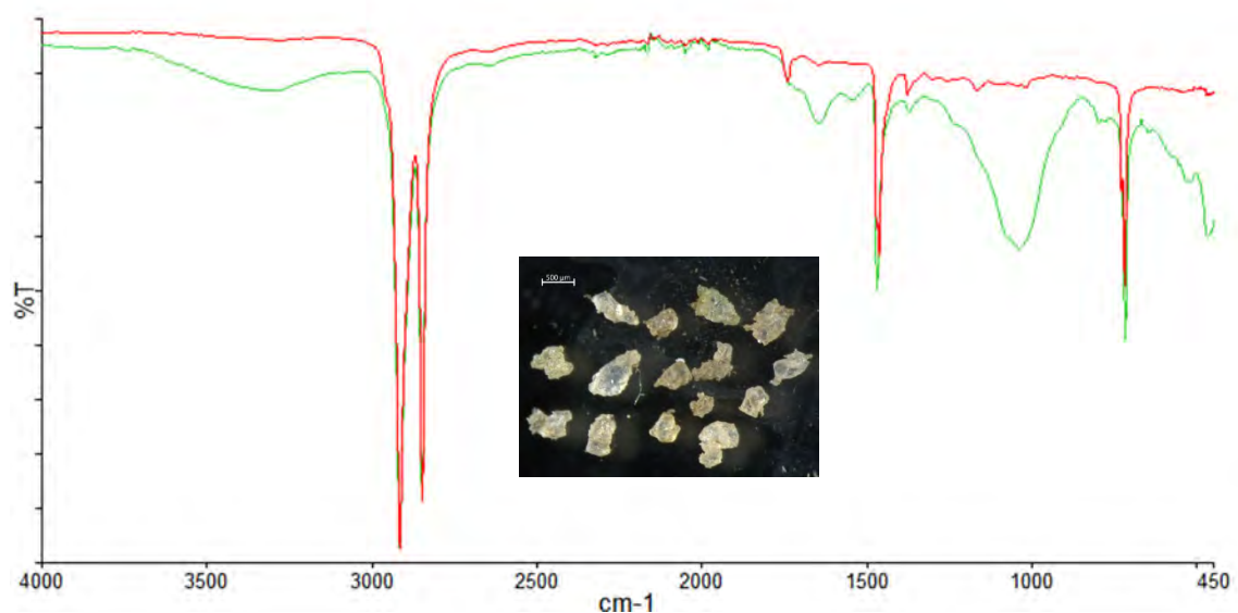
Figur 11. Partiklar från Svartåns utlopp, Hjälmaren, identifierade som polyeten (PE) med ATR-FTIR Grönt spektrum = partikel från Svartån. Rött spektrum = referensprov PE.
