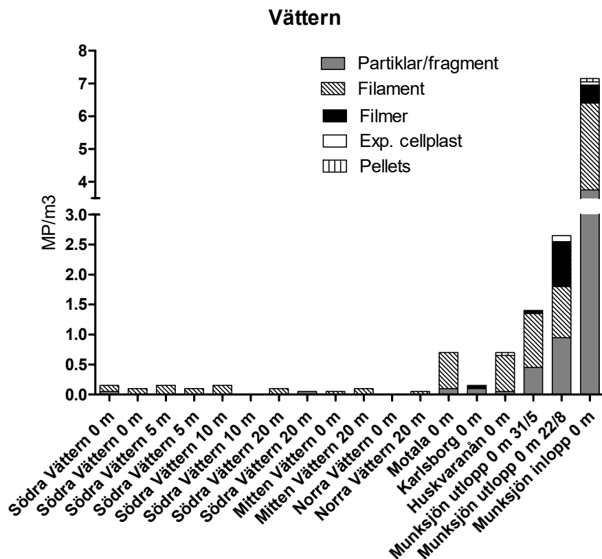
Figur 8. Sammansättning och antal mikroplaster > 300 µm (MP/m³) i proven från Vättern.
