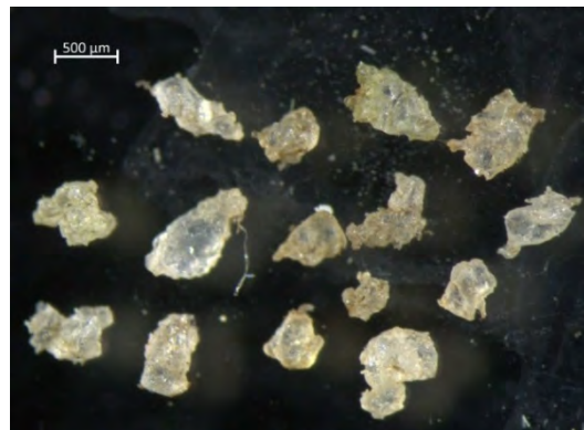
d) PE partiklar, Svartåns utlopp, Hjälmaren
