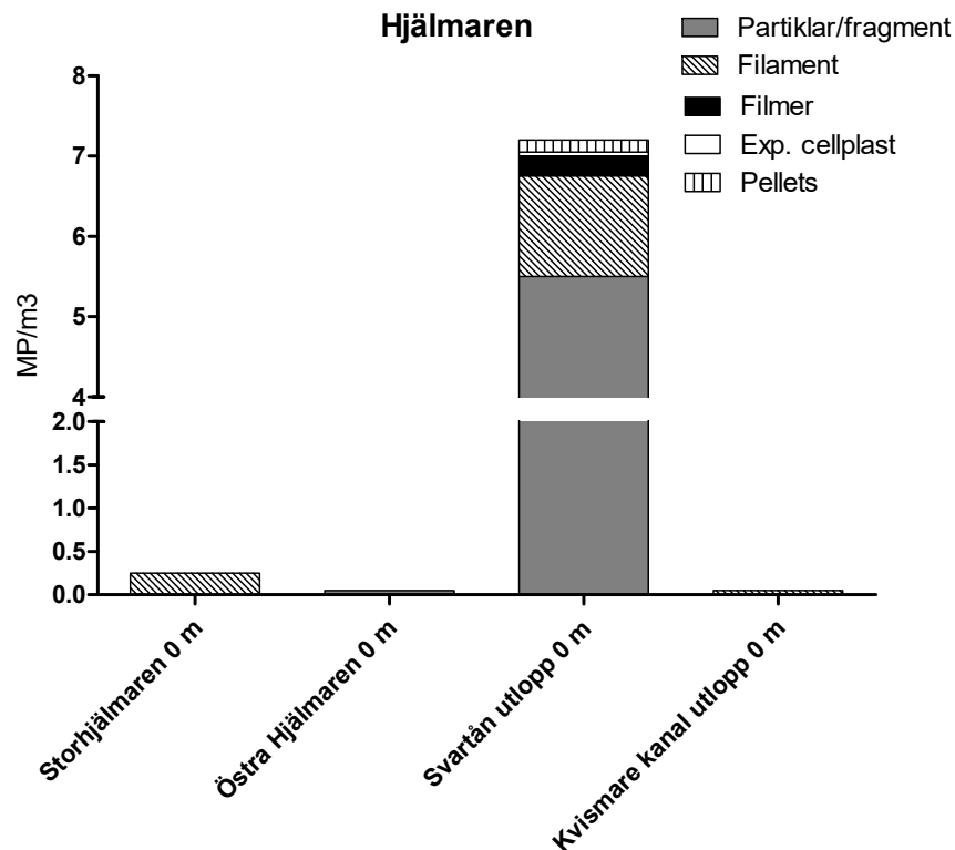
Figur 6. Ovan: Sammansättning och antal mikroplaster > 300 µm (MP/m³) i proven från Hjälmaren. Nedan: Provtagning i Hjälmaren.
