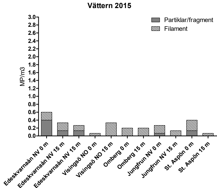
Figur 9. Sammansättning och antal mikroplaster > 300 µm (MP/m³) i proven från Vättern 2015.
