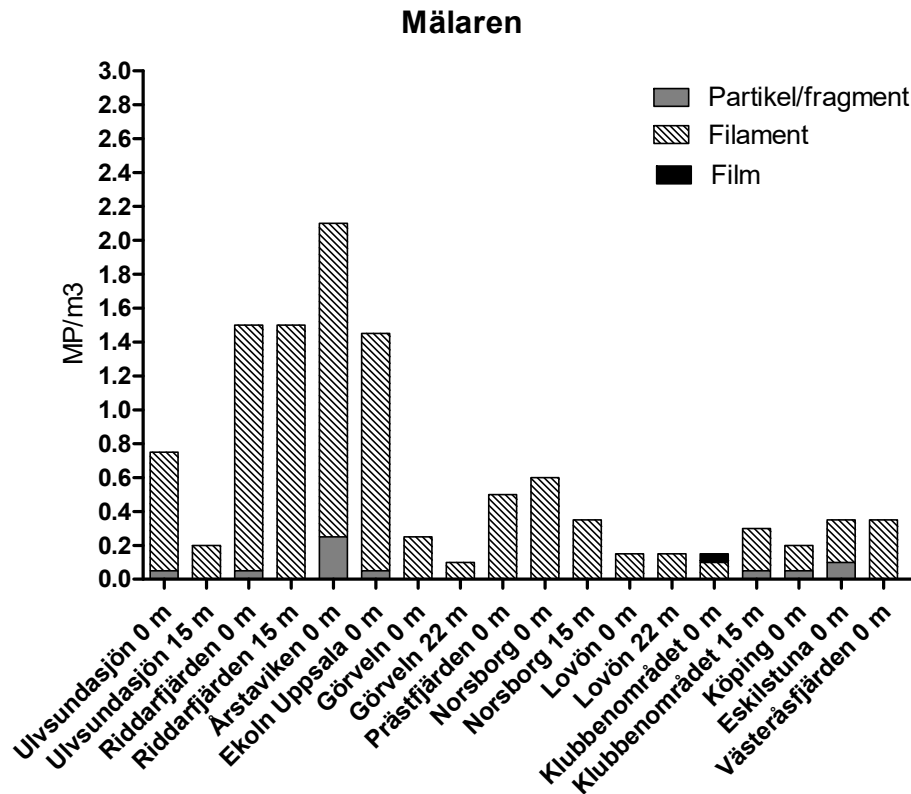
Figur 7. Sammansättning och antal mikroplaster > 300 µm (MP/m³) i proven från Mälaren.
