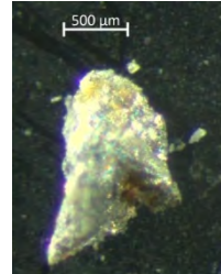
Metallisk partikel från Ulvsundasjön Mälaren.
